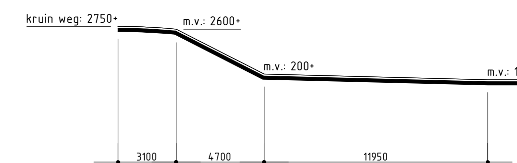
bestaande doorsnede A-A
