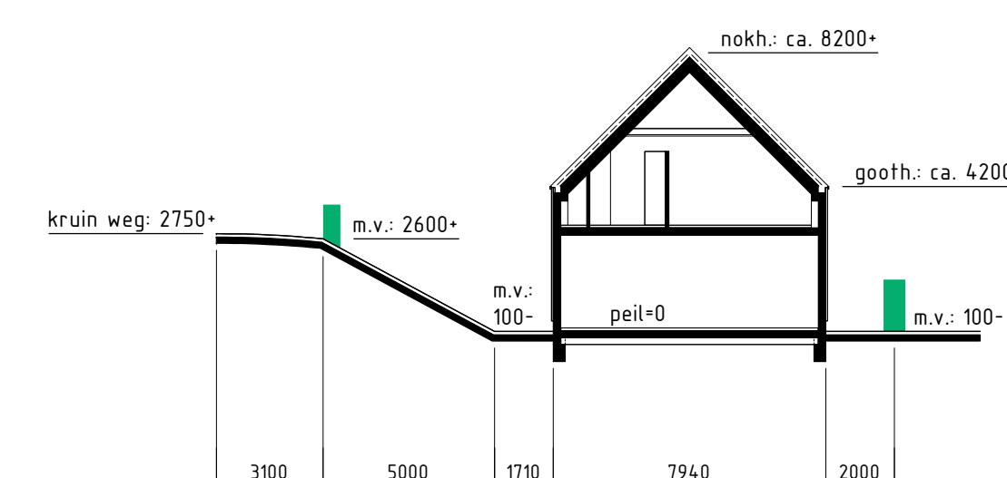
gewijzigde doorsnede A-A
