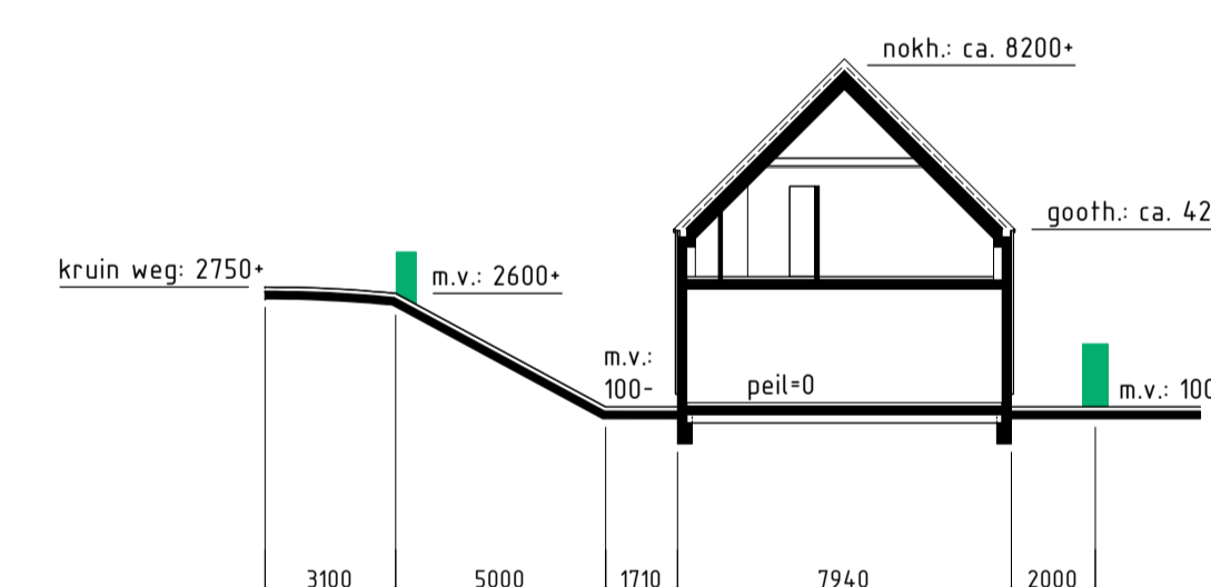
gewijzigde doorsnede A-A
