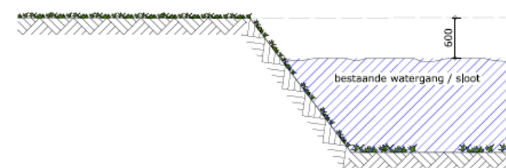
Doorsnede bestaande situatie
