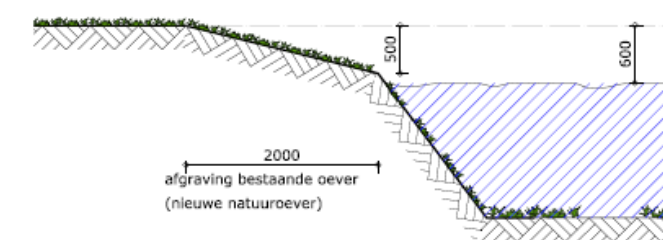
Doorsnede nieuw situatie
